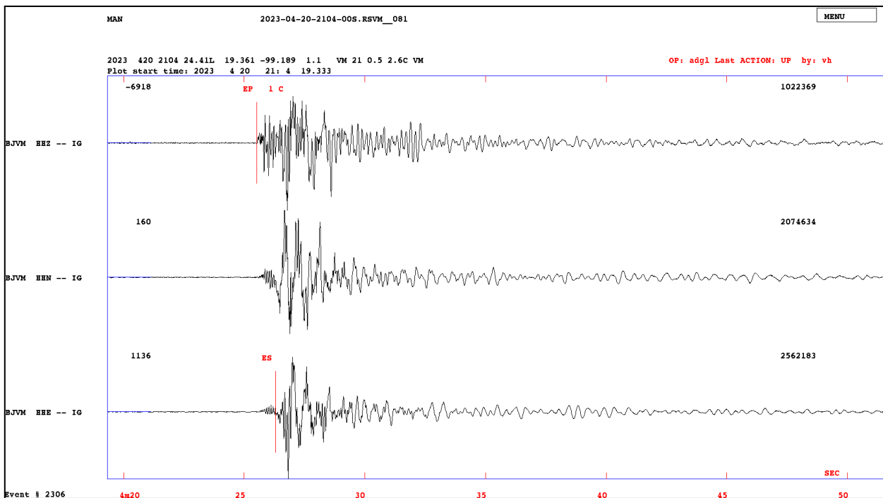
Figura 2. Registros sísmicos del evento del día 20 de abril de 2023, M 2.6.
