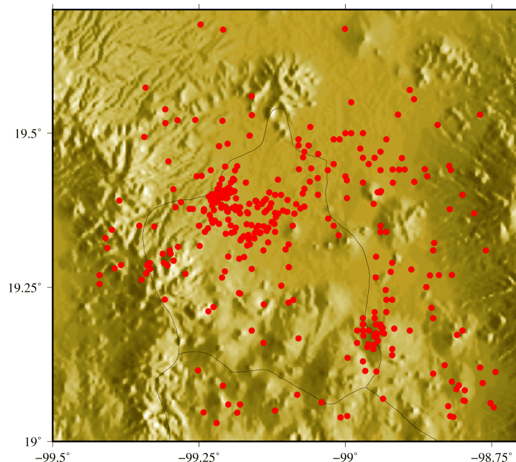
Figura 6. Sismos reportados por el Servicio Sismológico Nacional con epicentro en la Cuenca de México entre los años 2000 y 2023 (SSN, 2023). Las magnitudes de los sismos están entre 1.0 y 4.0.
