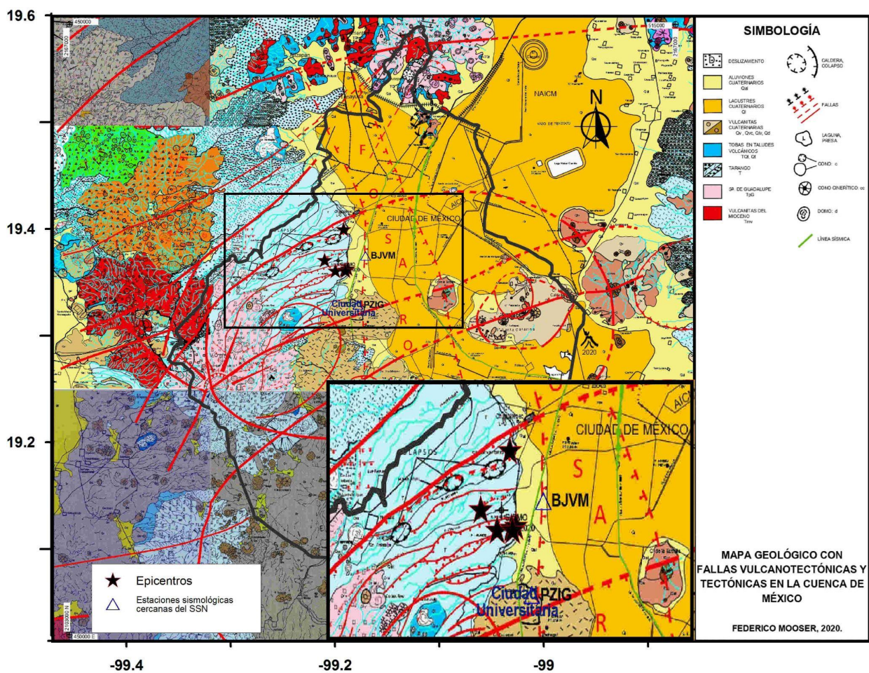
Figura 3. Ubicación de los sismos del 29 de marzo al 21 de abril de 2023, con epicentro en la Ciudad de México (estrellas negras). Se pueden ver las localizaciones epicentrales dentro del contexto del terreno y fallamiento existente en la Ciudad de México.
