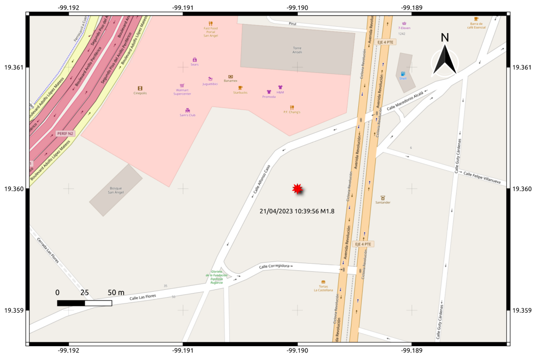
Figura 1. Epicentro del sismo del día 21 de abril de 2023.
