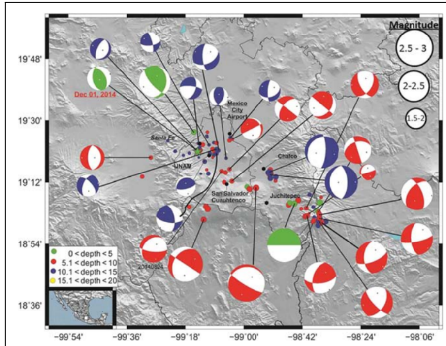
Figura 5. Sismicidad registrada por la Red Sísmica del Valle de México del SSN entre los años 2011 y 2017. El tamaño del mecanismo focal corresponde a la magnitud del sismo (Quintanar et al., 2018).
